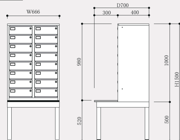
寸法図
